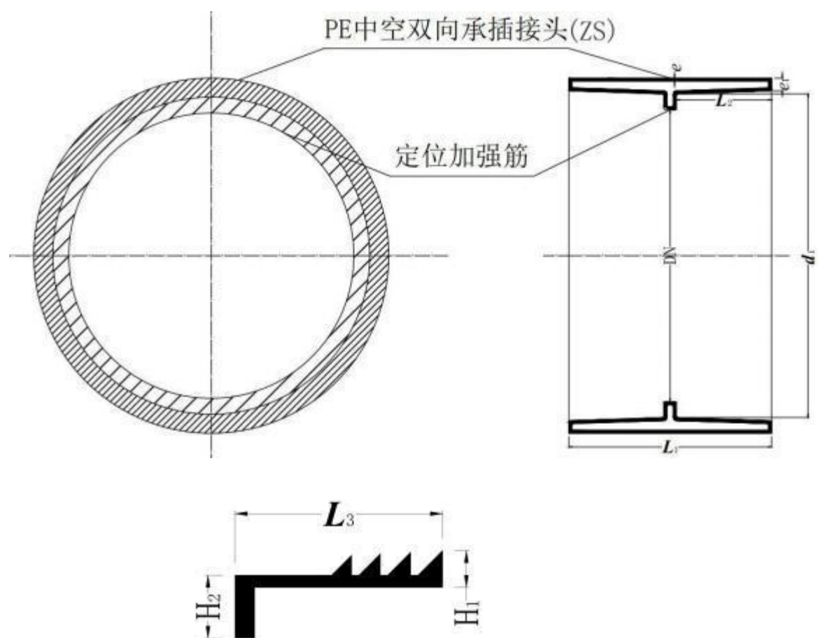
PE双向承插接头(ZS)及L形多峰橡胶密封圈
