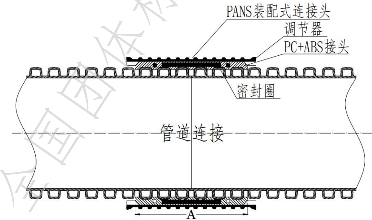
图 2 管材 PANS 装配式连接示意图
