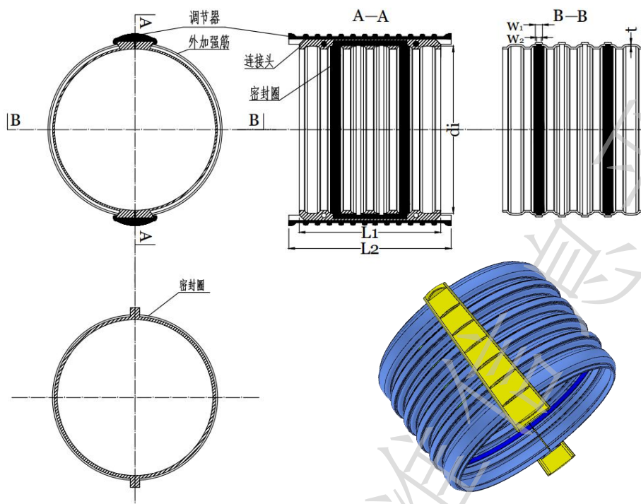
图3 PANS装配式连接头示意图
