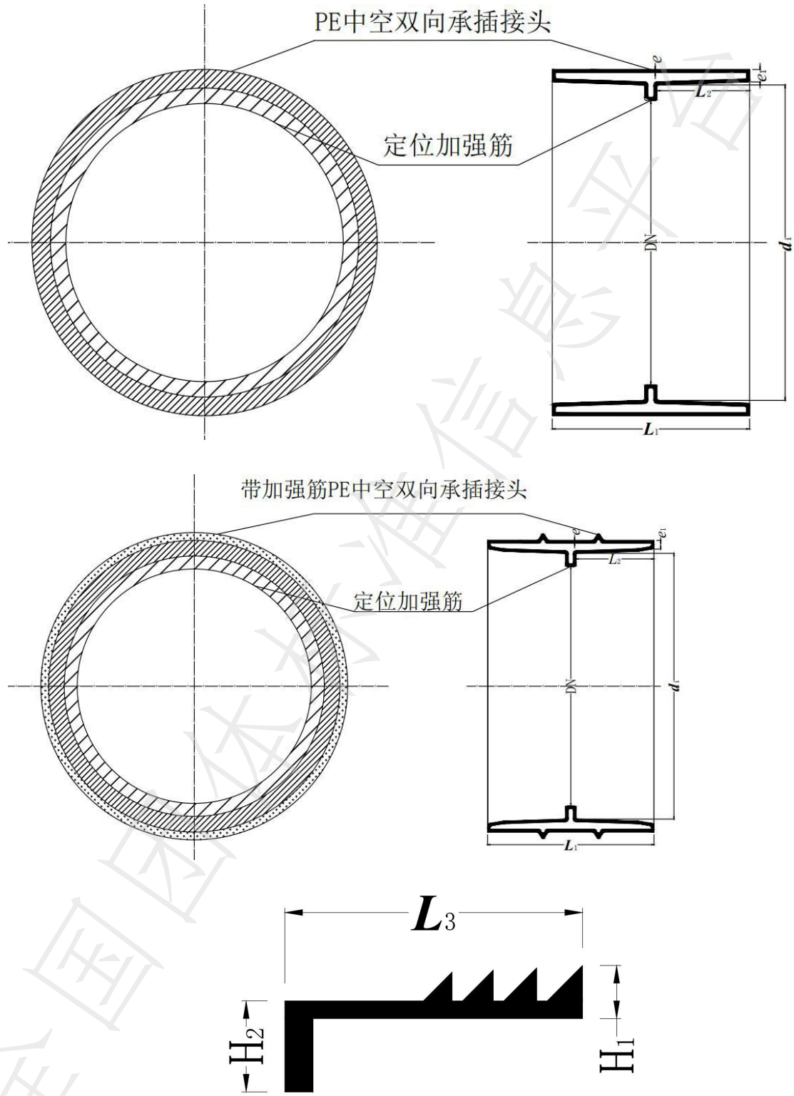
图3 PE双向承插接头及L形多峰橡胶密封圈
