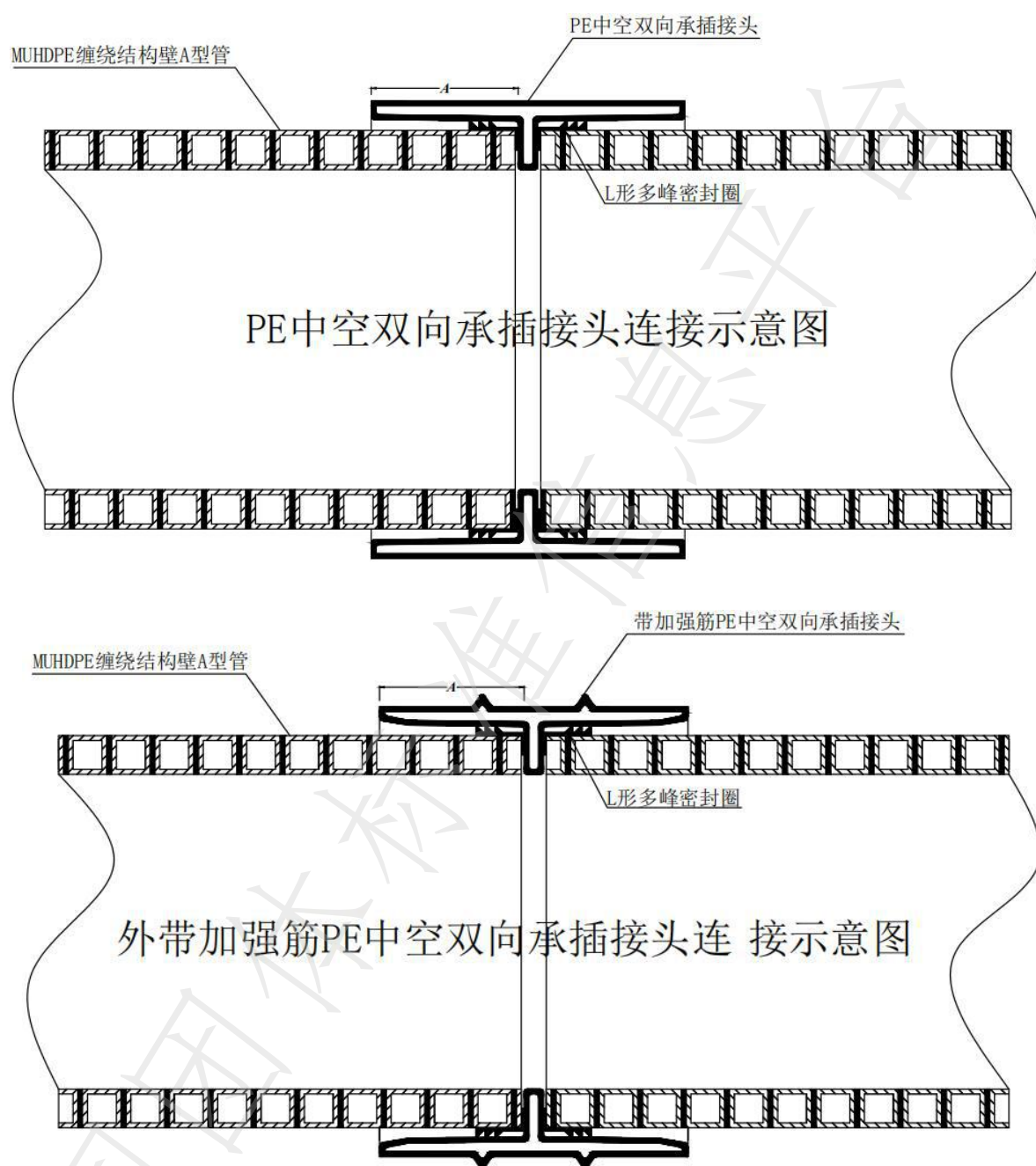
图2 管材双向承插连接示意图
