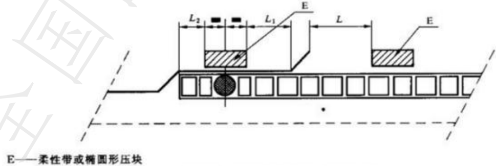
图 B. 3 在连接密封处压块的定位
