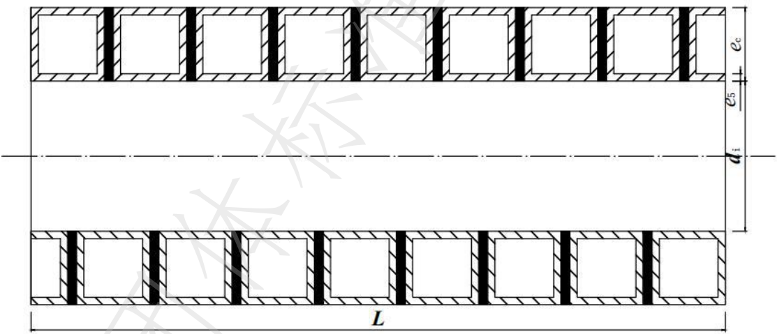
图 1 管材结构示意图
