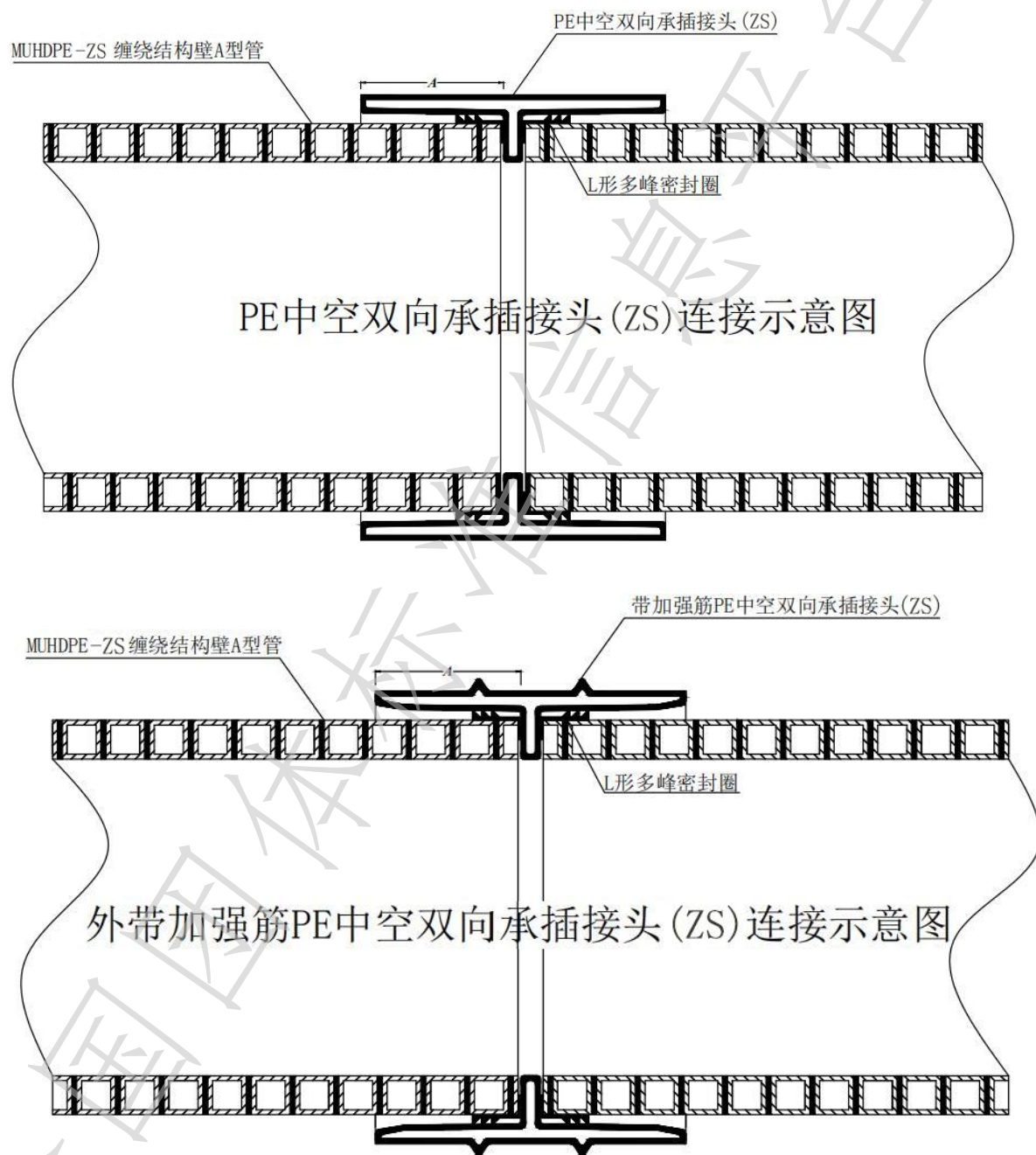
图2 管材中空双向承插接头（ZS）连接示意图
