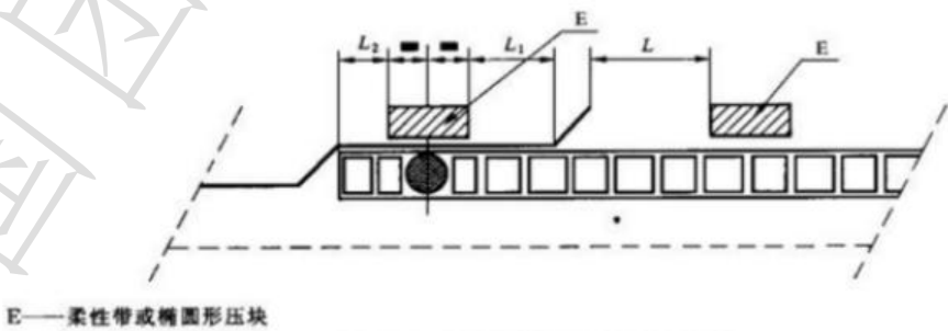
图 B. 3 在连接密封处压块的定位
