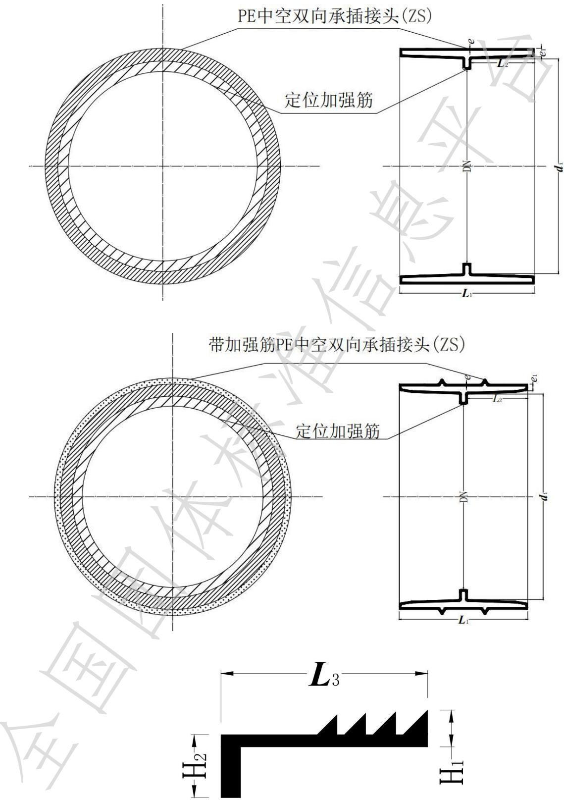
图3 PE中空双向承插接头 (ZS) 及L形多峰橡胶密封圈
