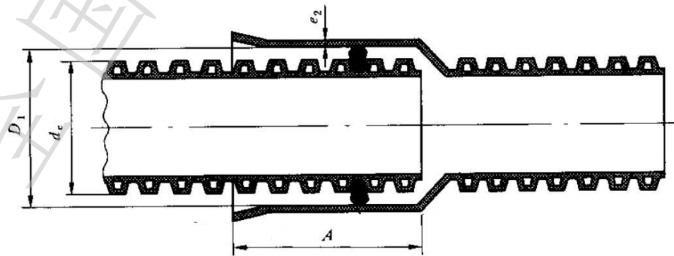
图 2 管材承插连接示意图
