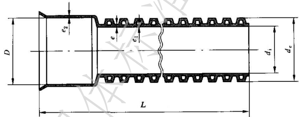
图 1 管材结构示意图
