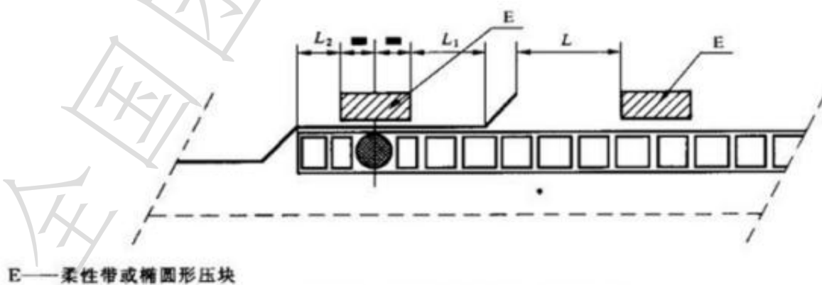
图 B.3 在连接密封处压块的定位
